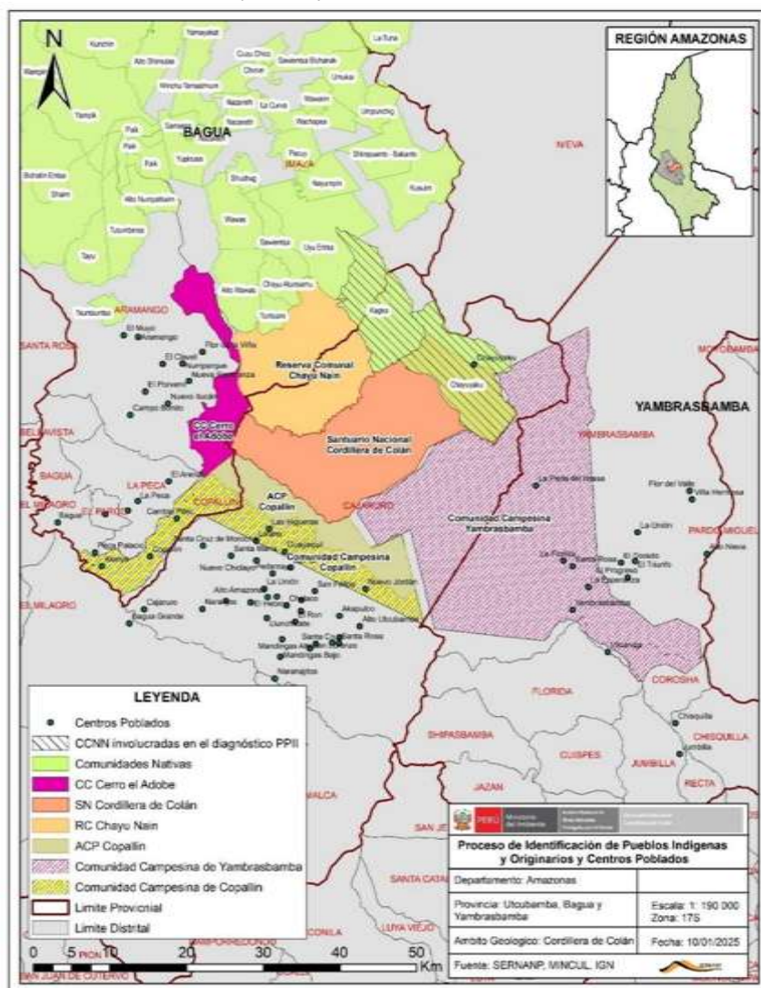
Figura 01: Ubicación del Santuario Nacional Cordillera de Colán
